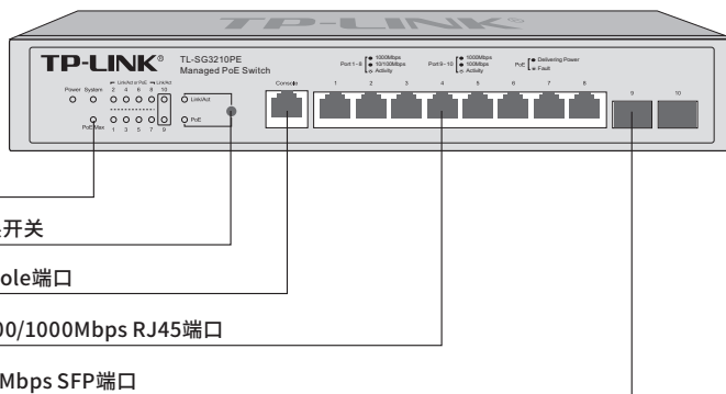
图1-10 TL-SG3210PE前面板示意图
