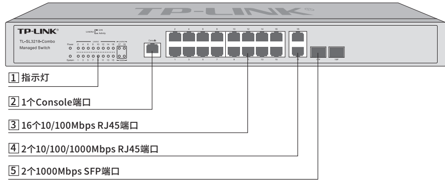
图1-15 TL-SL3218-Combo前面板示意图
